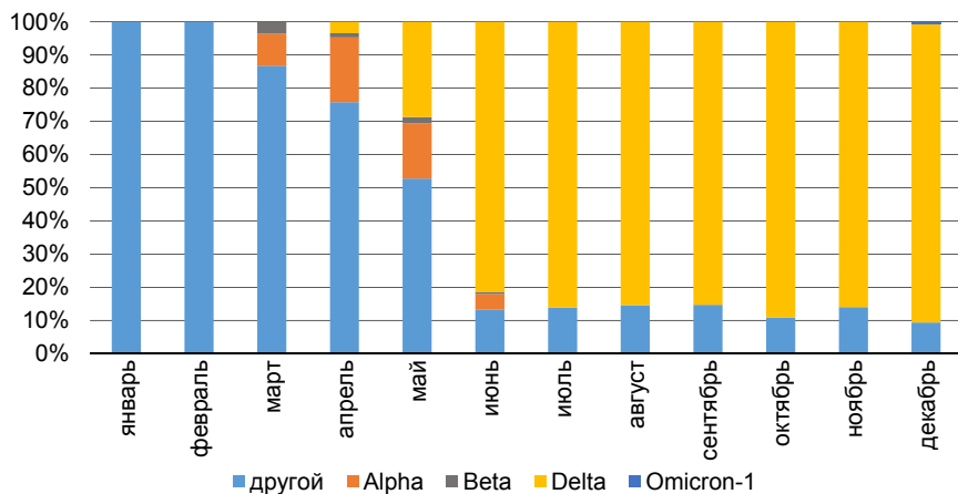
Рис. 32. Динамика идентифицированных геновариантов SARS-CoV-2 в субъектах СФО и ДФО в 2021 г.
